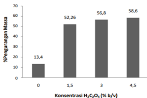
Gambar 1. Pengaruh Konsentrasi H 2 C 2 O 4 Terhadap Pengurangan Massa Pelepeh Nipah
